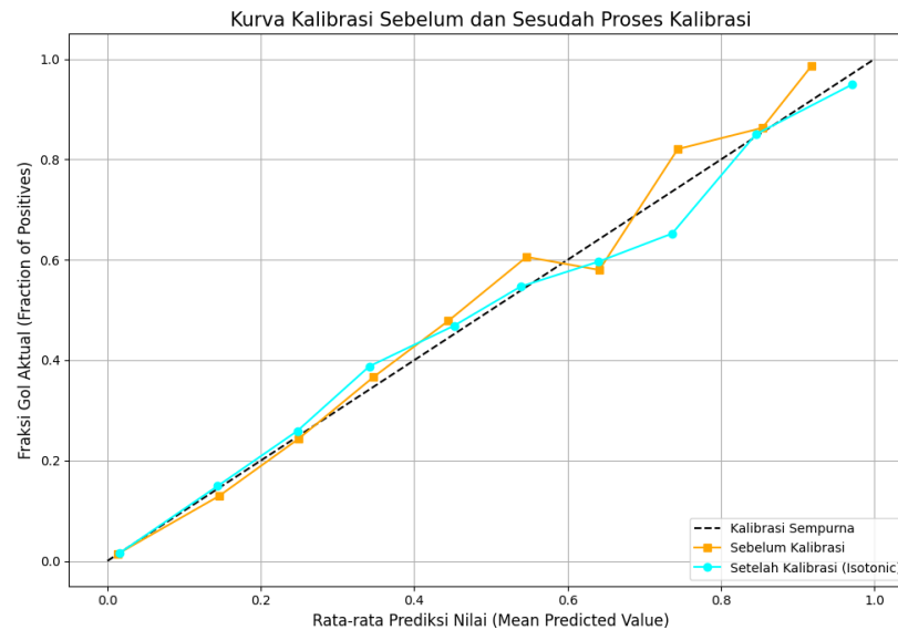
Gambar 4.25 Kurva Kalibrasi Sebelum dan Sesudah Proses Kalibrasi
