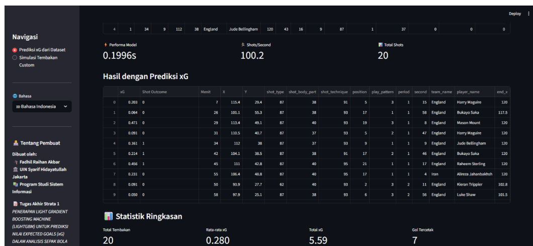
Gambar 4.29 Tampilan Halaman Prediksi Berdasarkan Dataset
